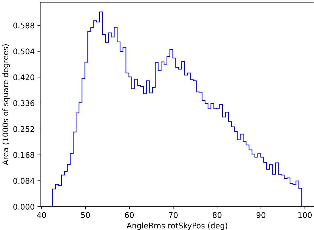
all_long_v3.4_10yrs All sky i band: AngleRms rotSkyPos
