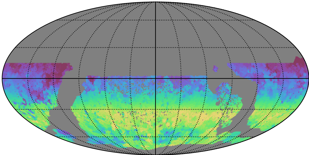
all_long_v3.4_10yrs WFD y band: AngleRange rotSkyPos
