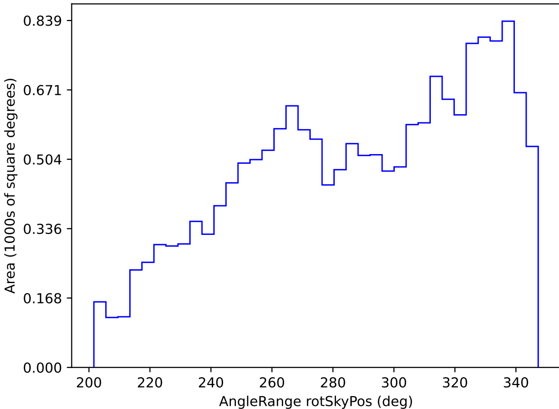
all_long_v3.4_10yrs WFD i band: AngleRange rotSkyPos
