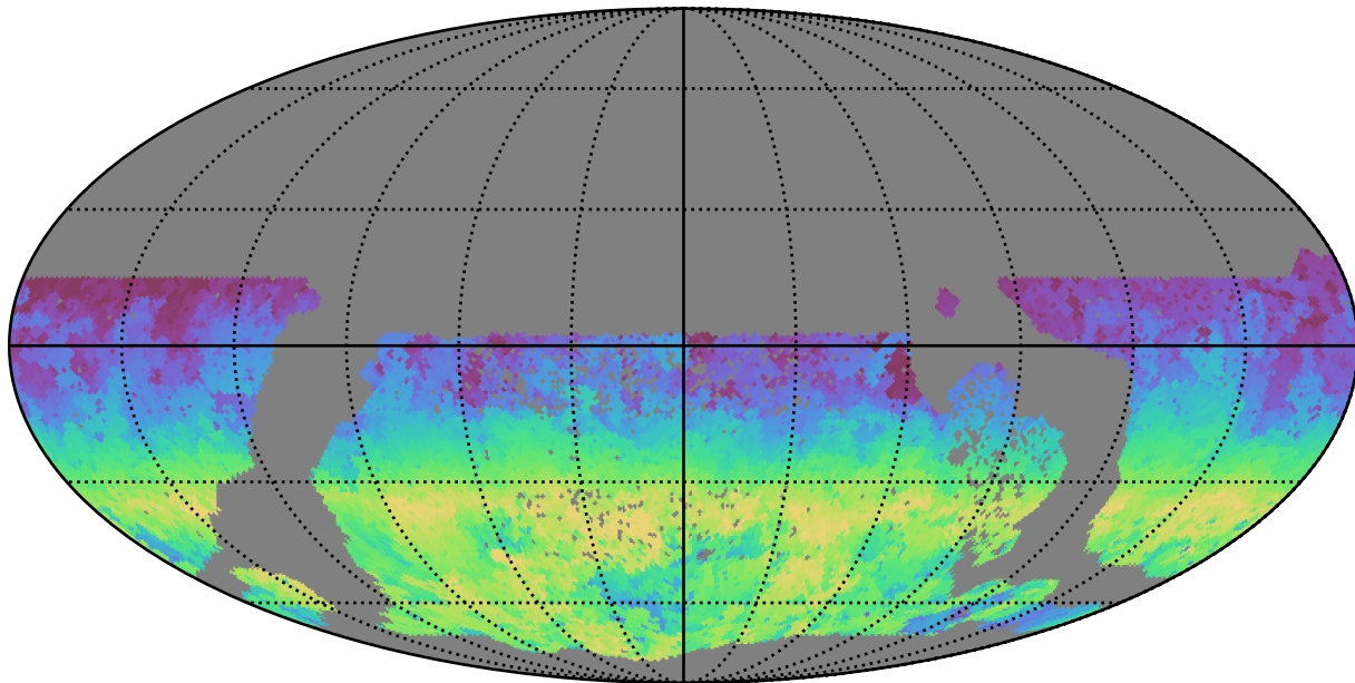
all_long_v3.4_10yrs WFD g band: AngleRange rotSkyPos
