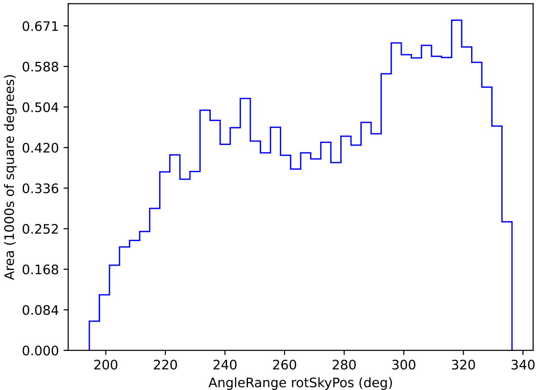
all_long_v3.4_10yrs WFD g band: AngleRange rotSkyPos
