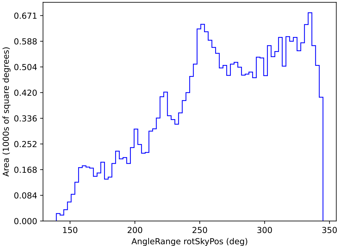
all_long_v3.4_10yrs All sky z band: AngleRange rotSkyPos
