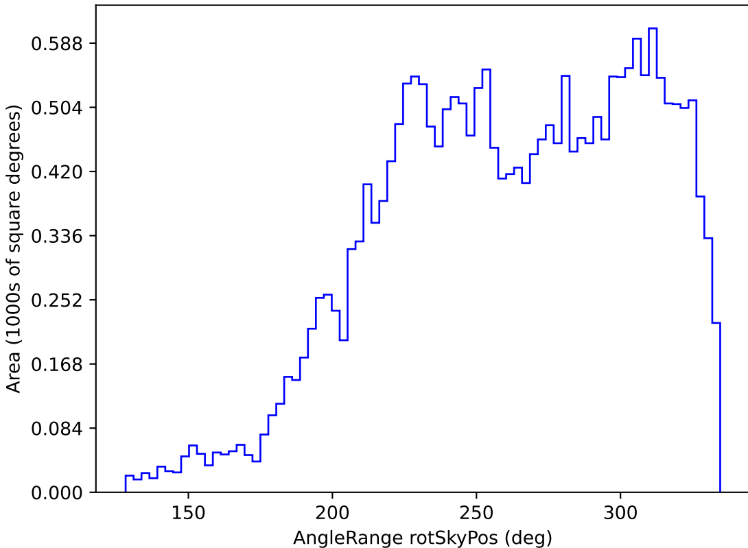
all_long_v3.4_10yrs All sky y band: AngleRange rotSkyPos
