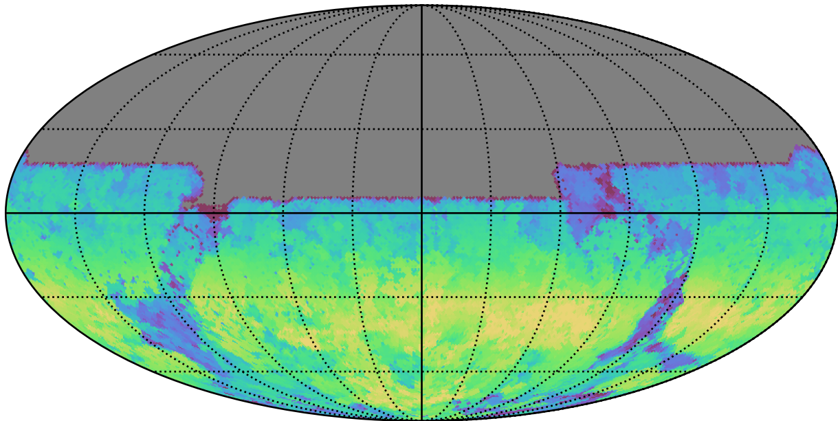
all_long_v3.4_10yrs All sky u band: AngleRange rotSkyPos
