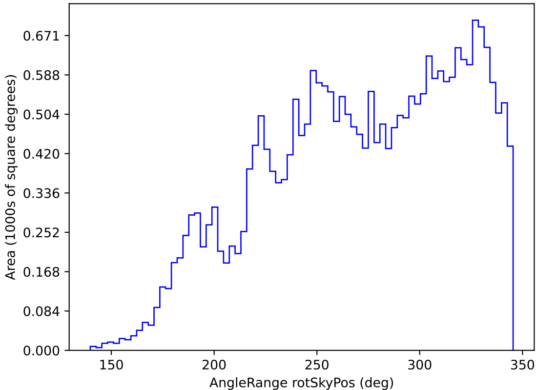
all_long_v3.4_10yrs All sky r band: AngleRange rotSkyPos
