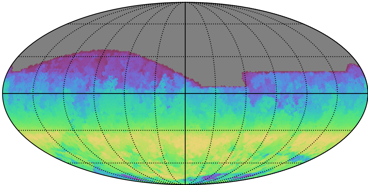
all_long_v3.4_10yrs All sky i band: AngleRange rotSkyPos
