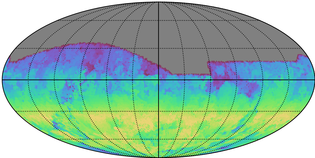
all_long_v3.4_10yrs All sky g band: AngleRange rotSkyPos
