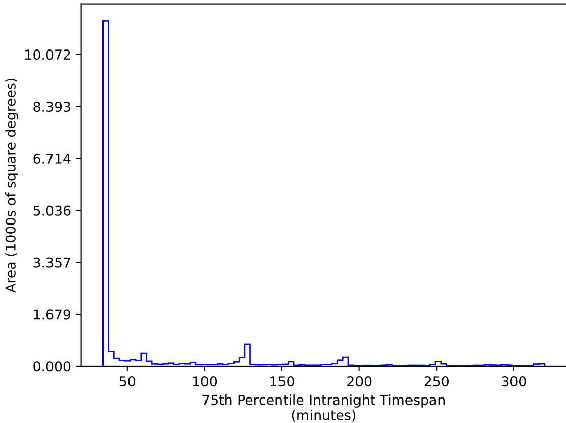
all_long_v3.4_10yrs WFD iz bands: 75th Percentile Intranight Timespan
