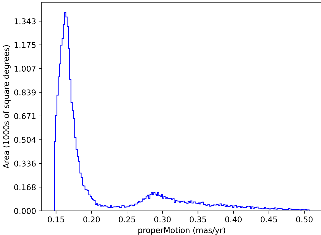
all_long_v3.4_10yrs : properMotion
