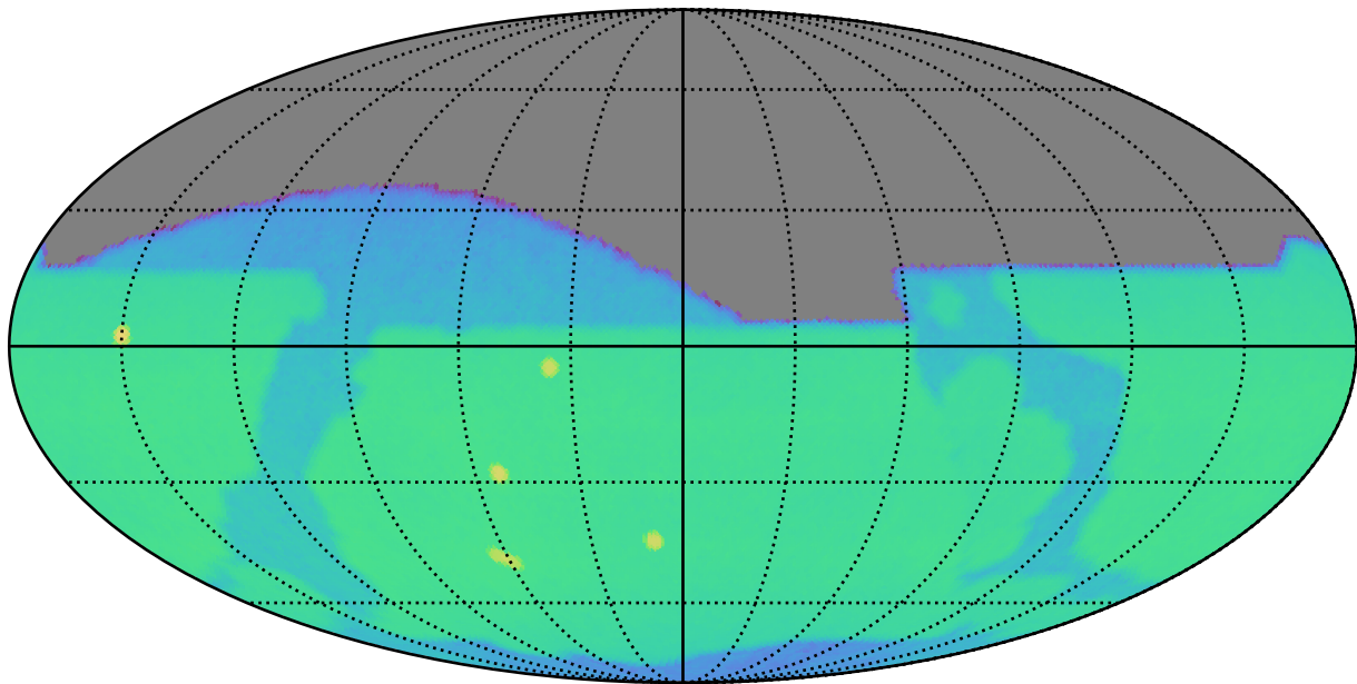
all_long_v3.4_10yrs z: CoaddM5
