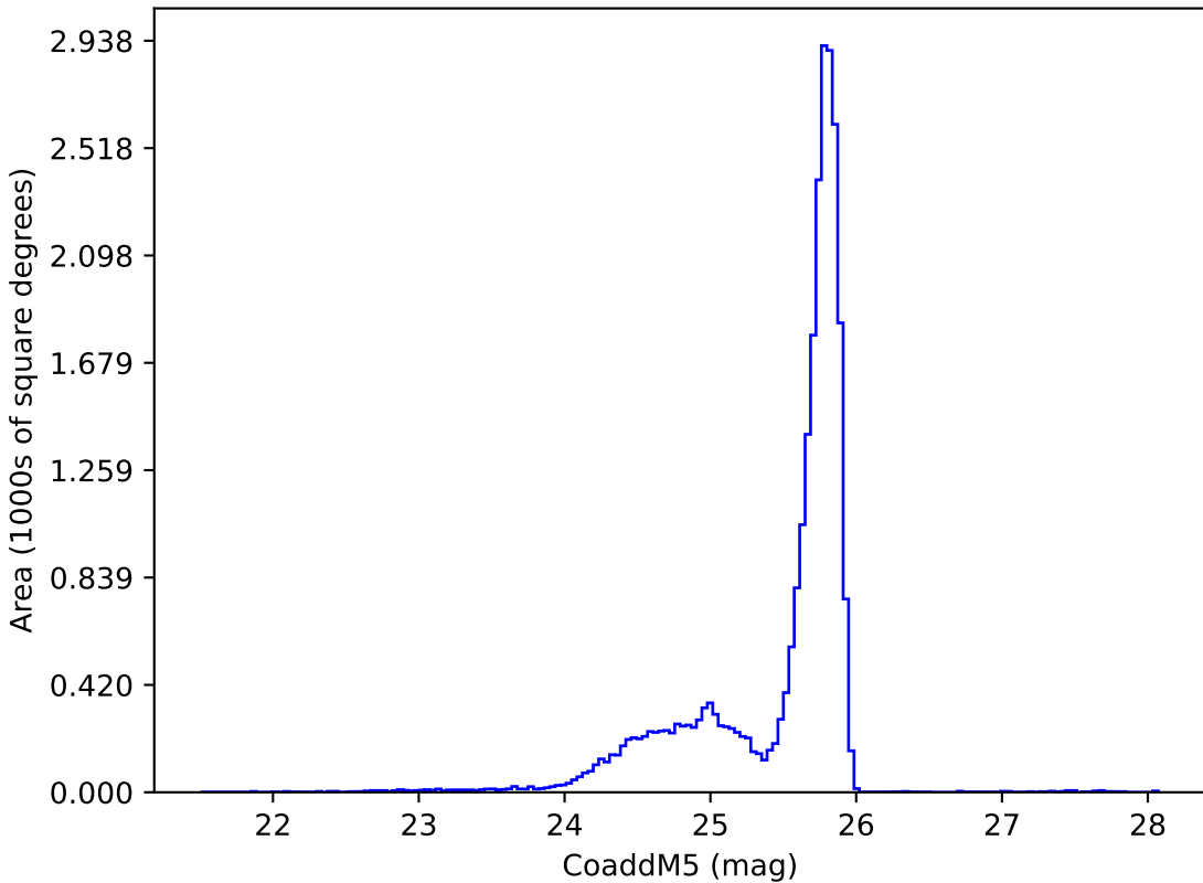
all_long_v3.4_10yrs z: CoaddM5
