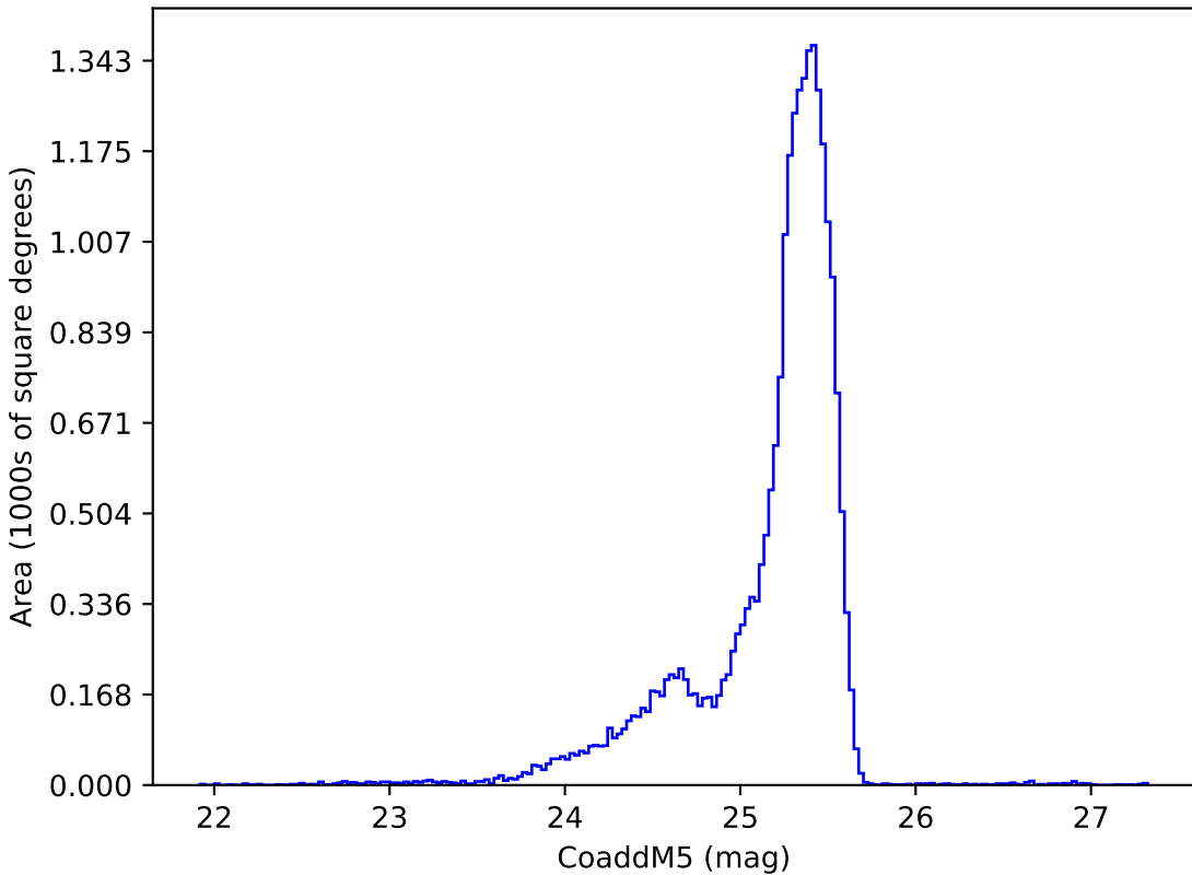
all_long_v3.4_10yrs u: CoaddM5
