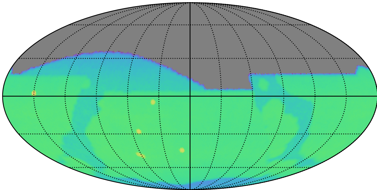
all_long_v3.4_10yrs r: CoaddM5
