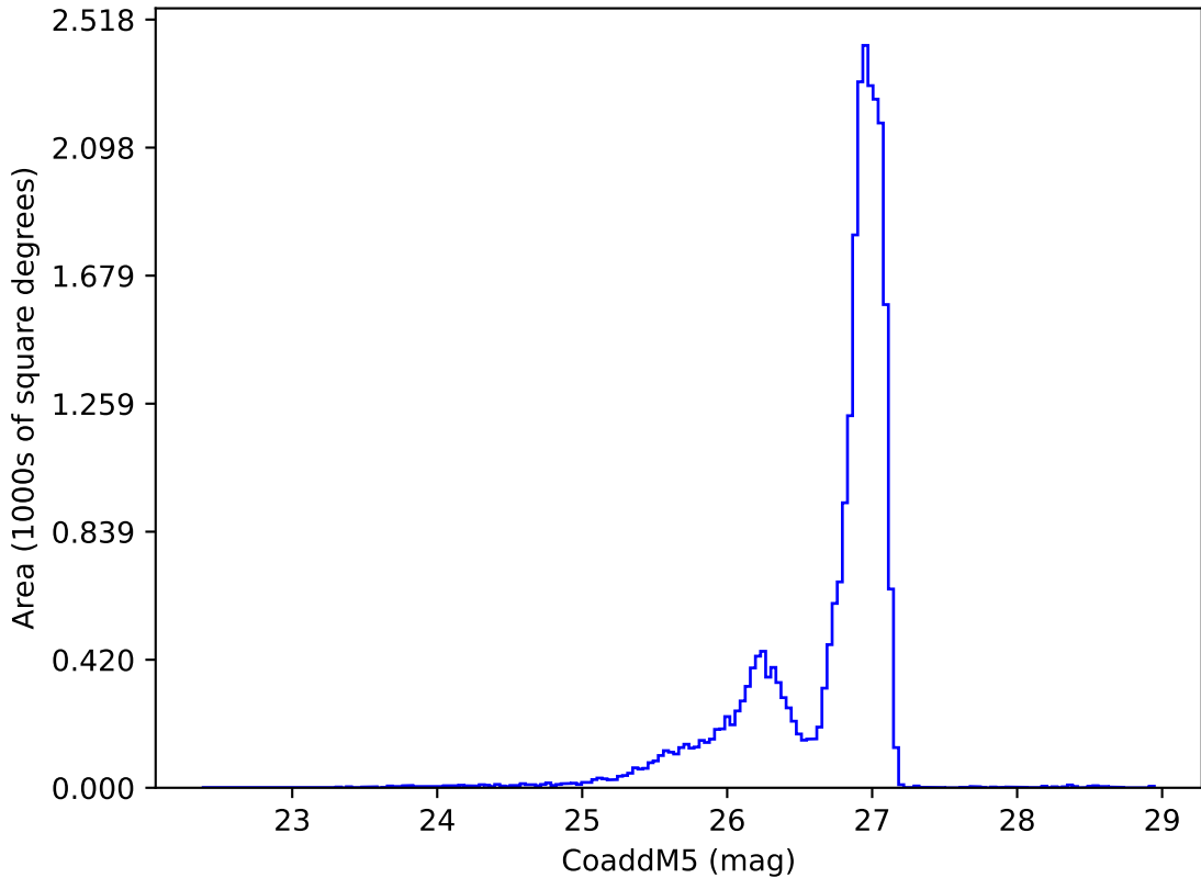
all_long_v3.4_10yrs r: CoaddM5
