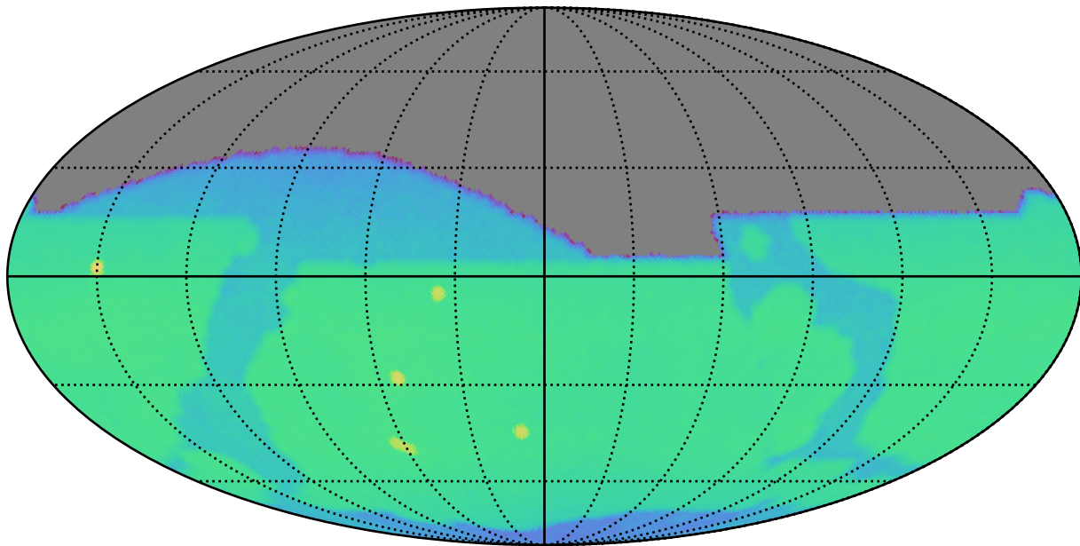
all_long_v3.4_10yrs i: CoaddM5
