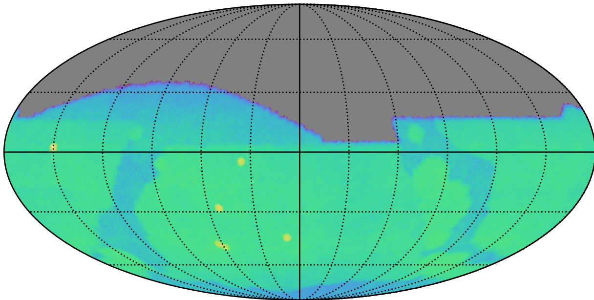
all_long_v3.4_10yrs g: CoaddM5
