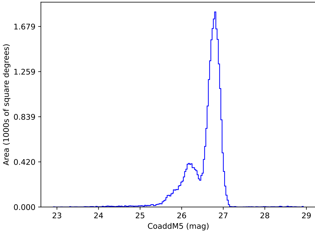
all_long_v3.4_10yrs g: CoaddM5
