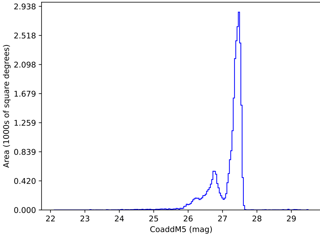
all_long_v3.4_10yrs : CoaddM5
