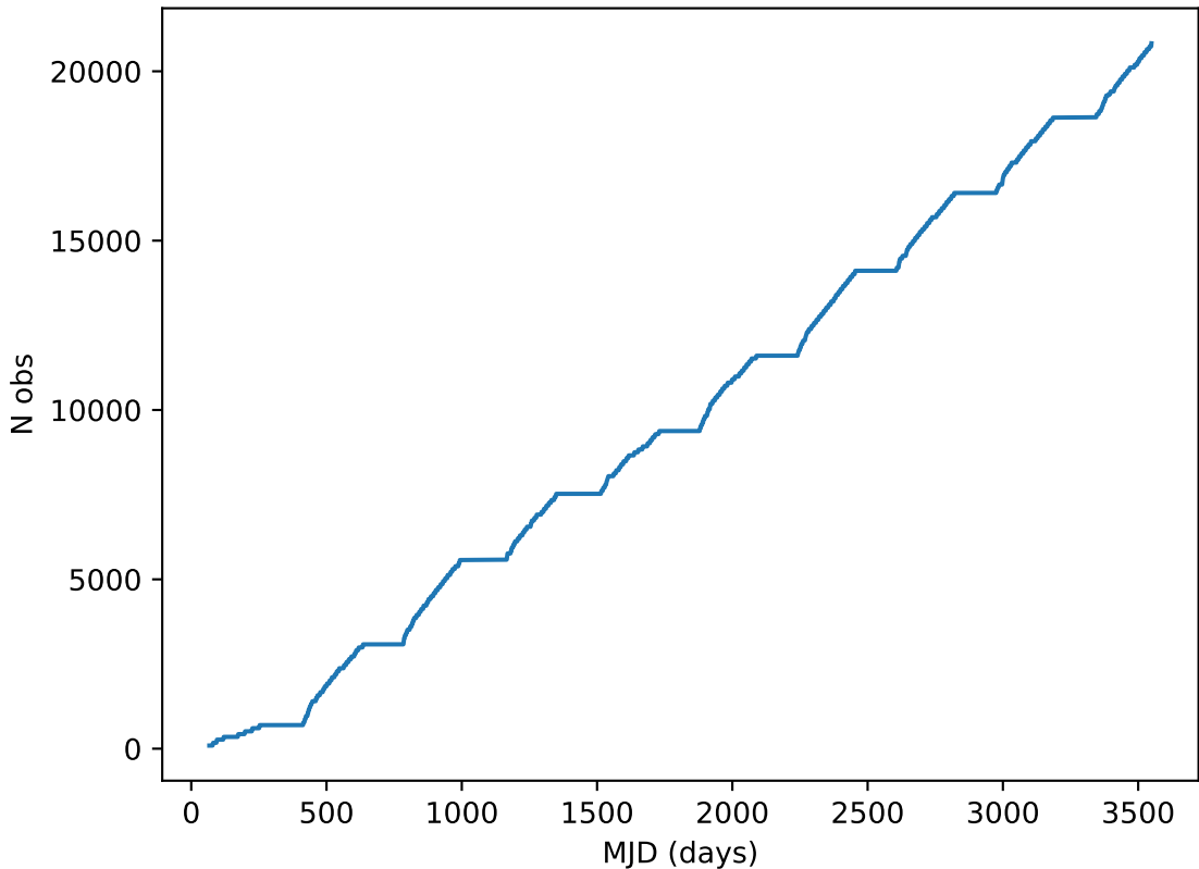
all_long_v3.4_10yrs all bands: DD:ELAISS1 Cumulative NVisits
