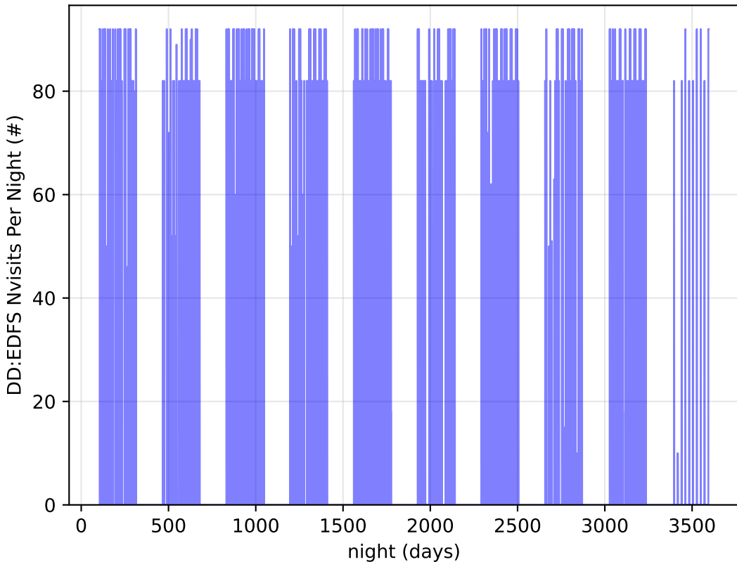
all_long_v3.4_10yrs all bands: DD:EDFS Nvisits Per Night
