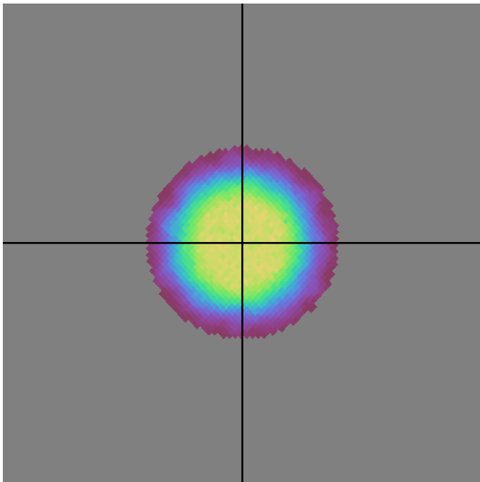
all_long_v3.4_10yrs g band: DD:ECDFS NVisits
