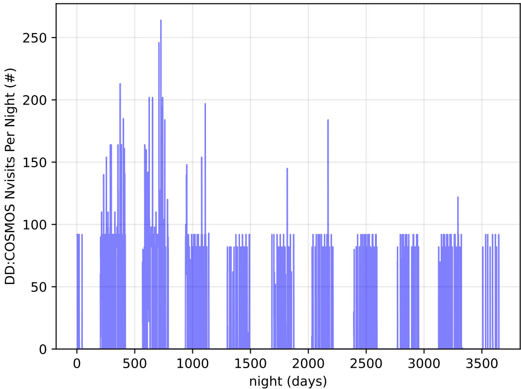
all_long_v3.4_10yrs all bands: DD:COSMOS Nvisits Per Night
